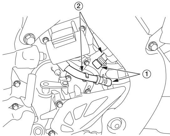
(1) крышки патрубков вентиляционной трубки картера (2) патрубки вентиляционной трубки картера
